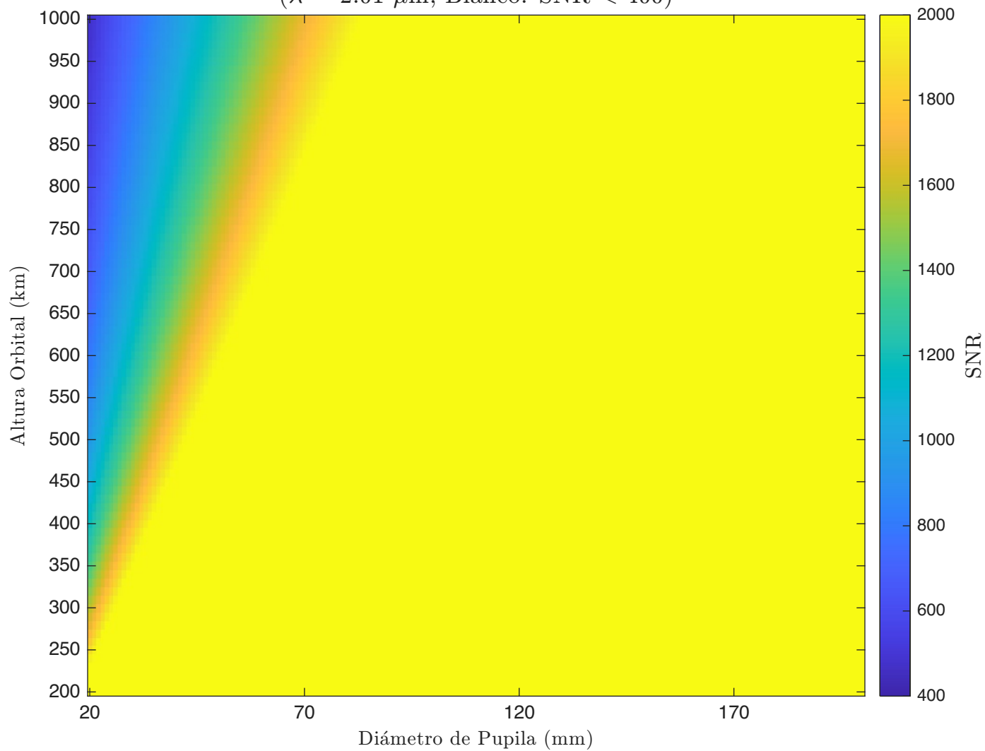
SNR - Refractivo - Detector 1 ( \lambda = 2.01 \mu\text{m} , Blanco: SNR < 400)
